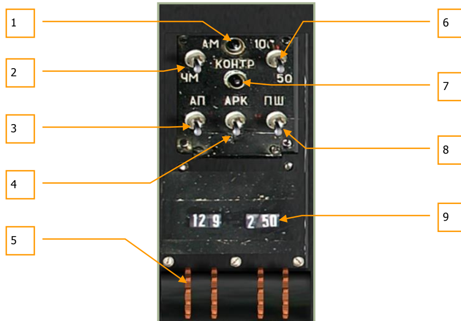
6-74: R-800L1 Funkgerätbedienpanel
