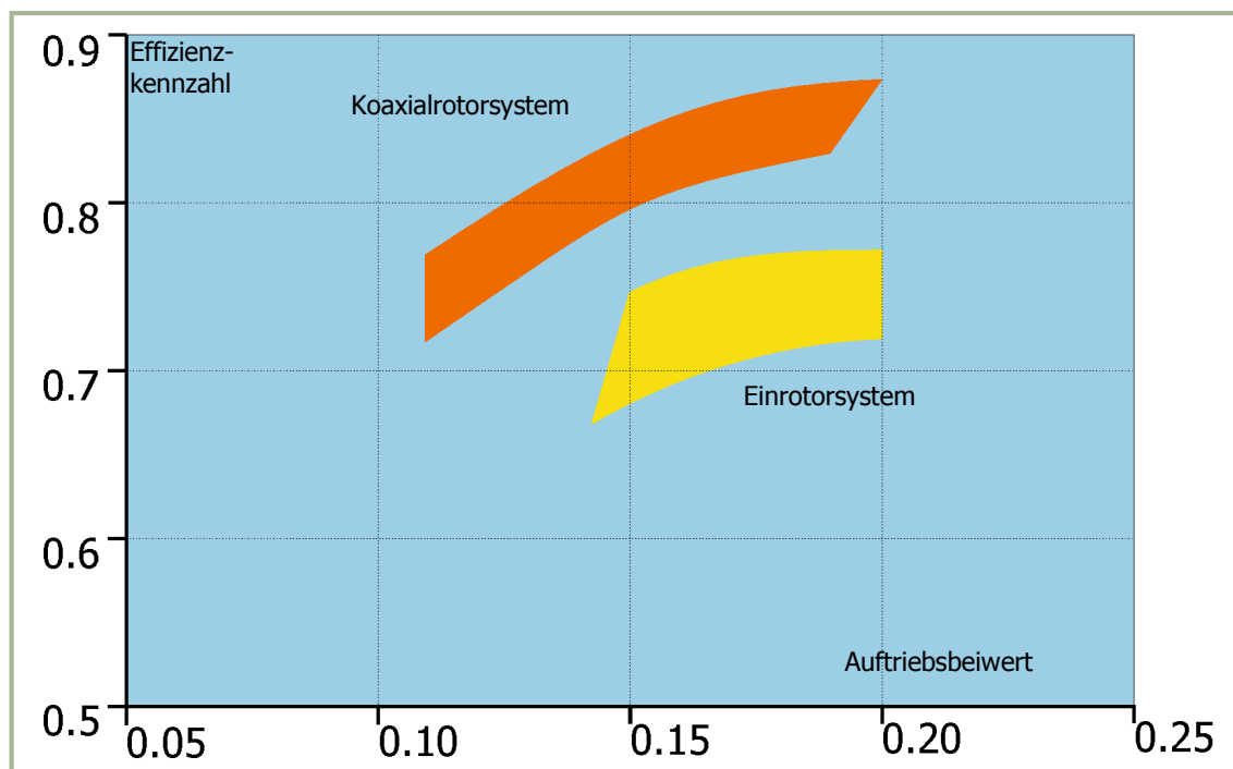
5-1: Vergleich der Schwebeflugeigenschaften von koaxialen und Einrotor-Systemen.
