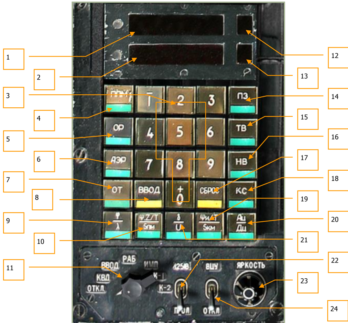
6-43: PVI-800 Panel für Navigationssteuerung
