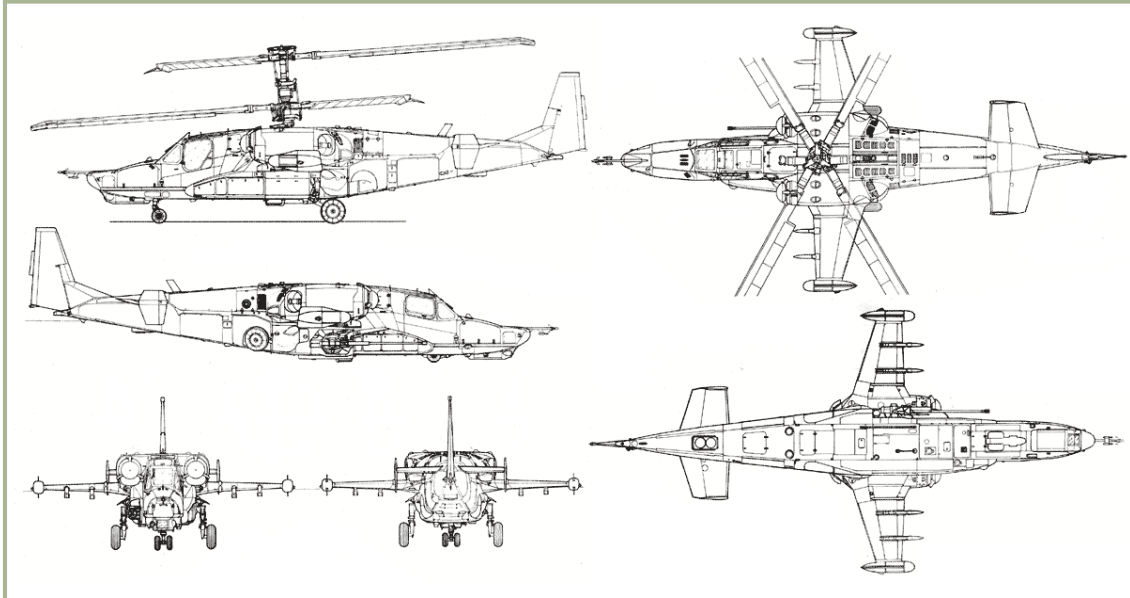
2-1: Ka-50 Zeichnungen
