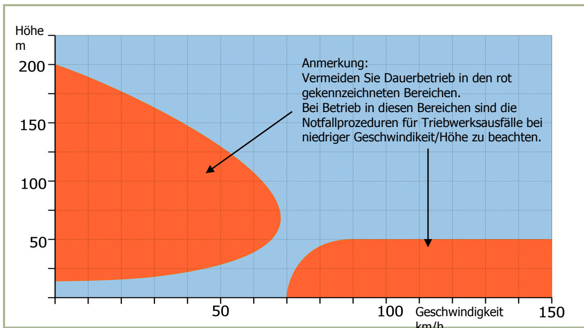
4-20: Höhen–Geschwindigkeits-Diagramm
