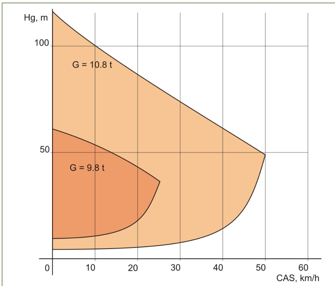
13-1: Kritische Flughöhen-Geschwindigkeits-Zone
