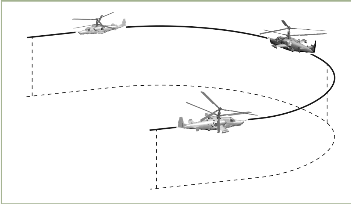
10-16: Flat yaw turn (Flache Kurve durch Gieren)
