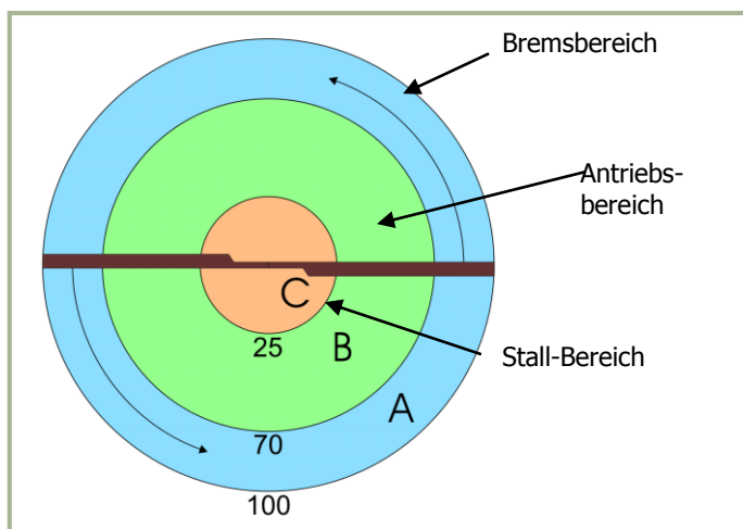
4-18: Rotorblattbereiche bei
