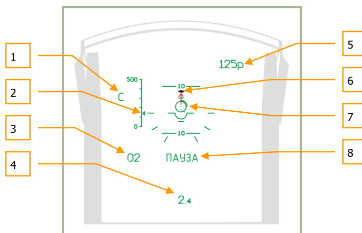
11-12: HUD Anzeigen beim Einsatz von Raketen oder fixierter Kanone ohne automatische Zielverfolgung
