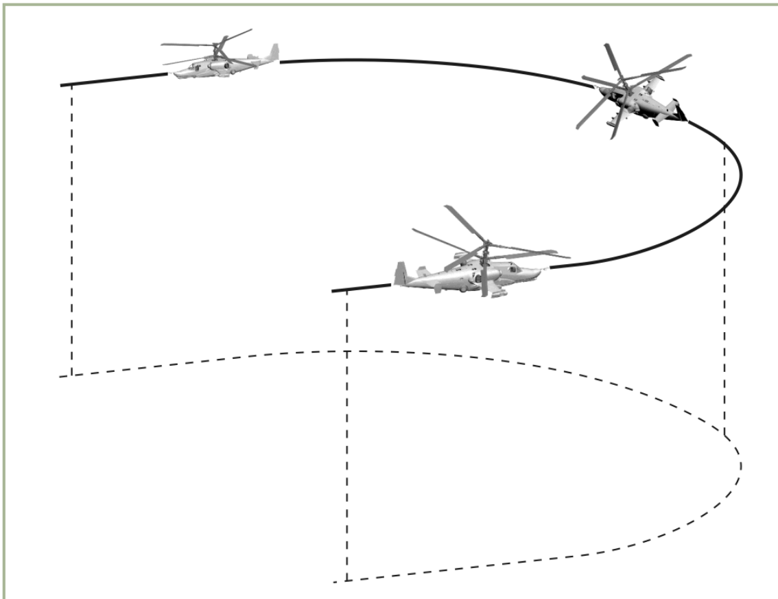
10-10: Koordinierte Kurve
