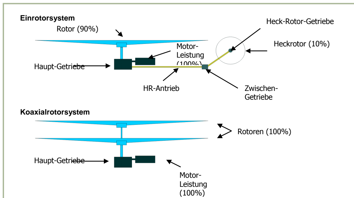
5-3: Coaxialer und konventioneller Rotorantrieb im Größenvergleich
