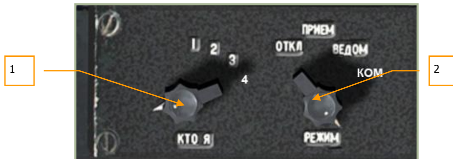
6-44: PVTz-800 Panel für die externe Zieldatenübertragung via Data Link
