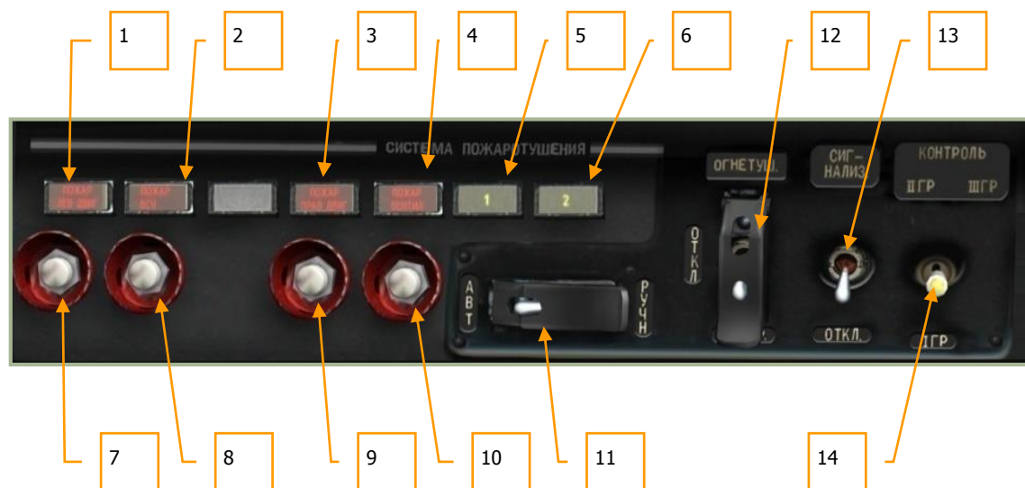
6-55: Feuerlöscher Kontrollpanel
