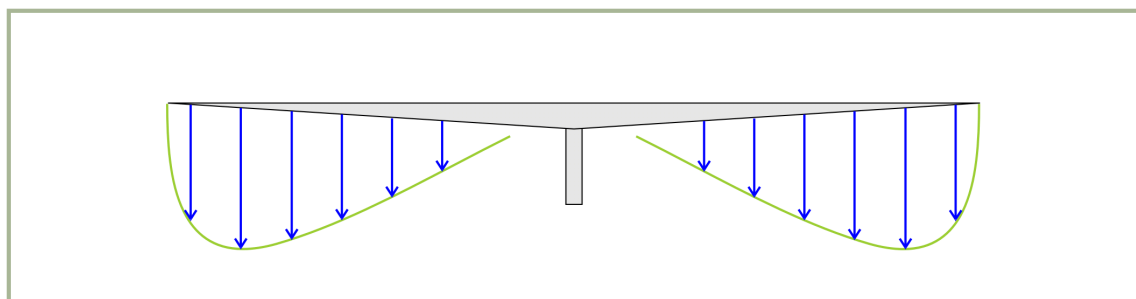
4-11: Induzierte Strömungsgeschwindigkeit im Schwebeflug
