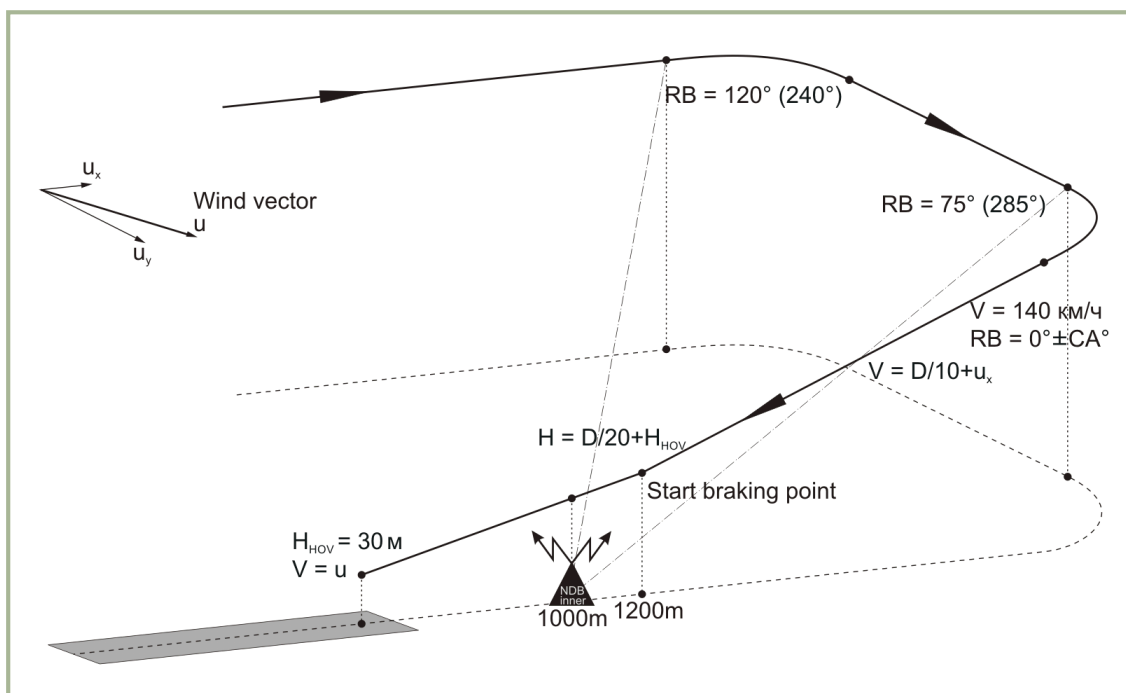
10-4: NDB Instrumentenanflug
